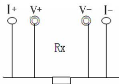
(a) 四端子接线图
