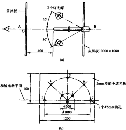
图4 检测可视指示,清晰可辨性的试验布置 (a) 俯视图; (b) 前板的正视图
