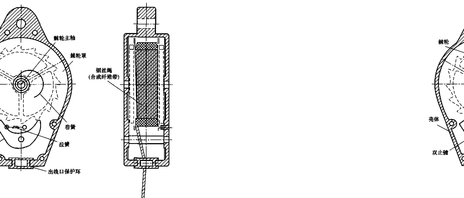
速差式防坠器典型结构和主要零部件示意图
