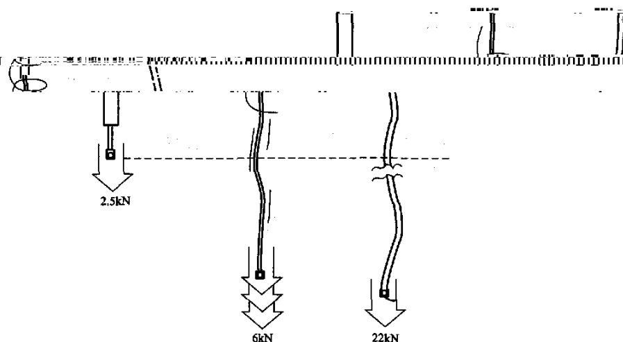
图 7 织带型缓冲器承载示意图
