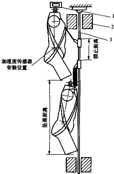
图 A.2 导轨式防坠器试验布置图
