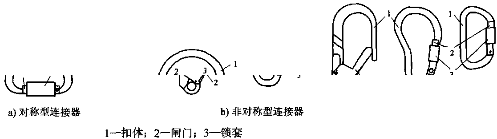
图3 连接器结构示意图
