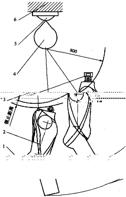
图 A.1 速差式防坠器试验布置图
